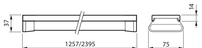
IP54-Lichtträger LL612X.../LL623X...
