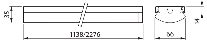
Lichtträger LL512X...PCO.../LL523X...PCO...
