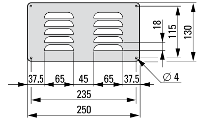
LVP-30H15-CS
