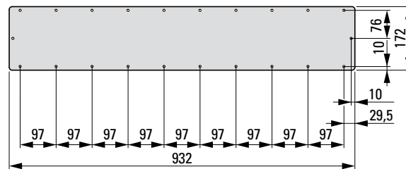
SFP-172X932-CS
