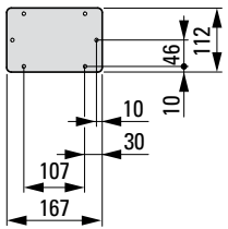
SFP-112X182-CS
