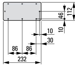
SFP-112X232-CS
