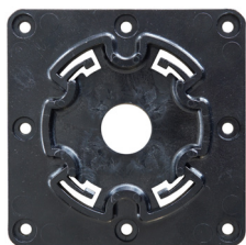
Art. 212121 Kunststoff-Clipslager 100x100mm; für Motoren bis 20Nm
