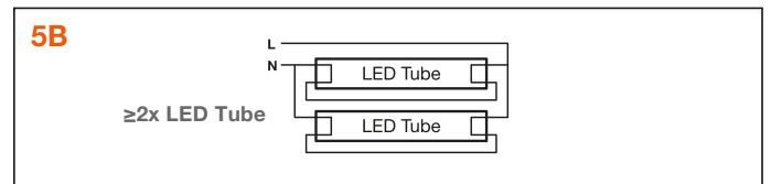
Umverdrahtung gemäß Verdrahtungsschema für mehrflammige Leuchten
