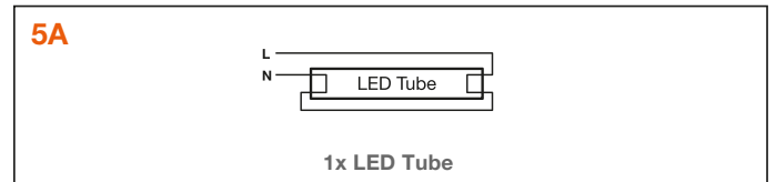
Umverdrahtung gemäß Verdrahtungsschema für einflammige Leuchten
