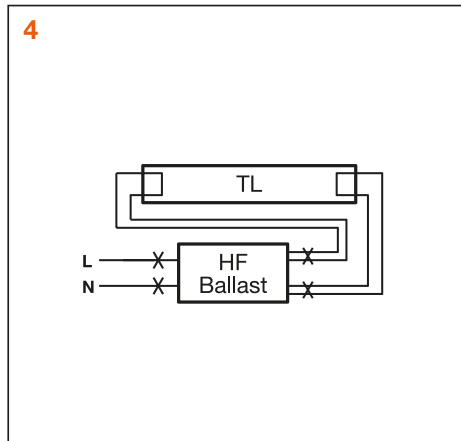
EVG/KVG/VVG aus der Leuchte entfernen Bei KVG/VVG: Kondensatoren zur Blindleistungskompensation ebenfalls entfernen
