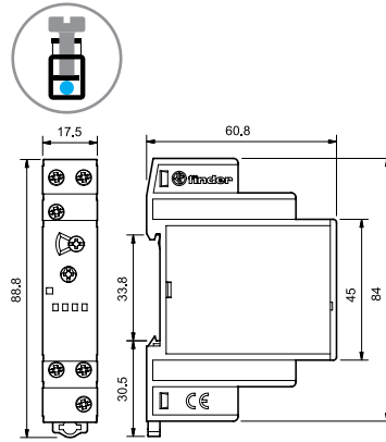
80.71 Schraubklemmen
