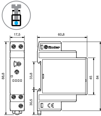
80.91 Schraubklemmen
